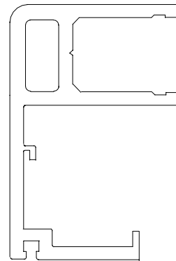
interlock stile FA 1046
